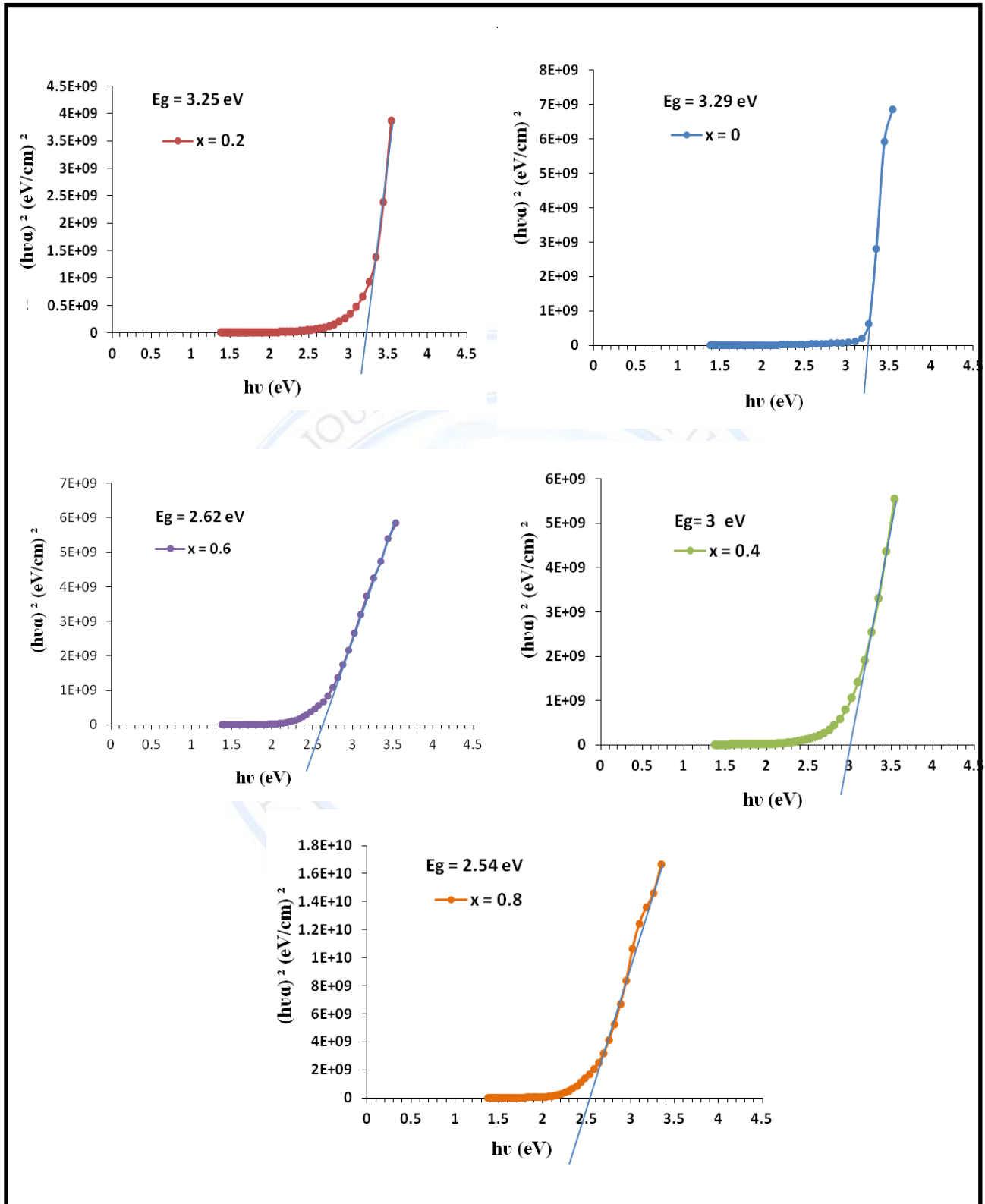
الشكل (٤): يوضح فجوة الطاقة البصرية لأغشية (Zn 1-x Fe x O) بالنسب الحجمية (x = 0, 0.2, 0.4, 0.6, 0.8).
