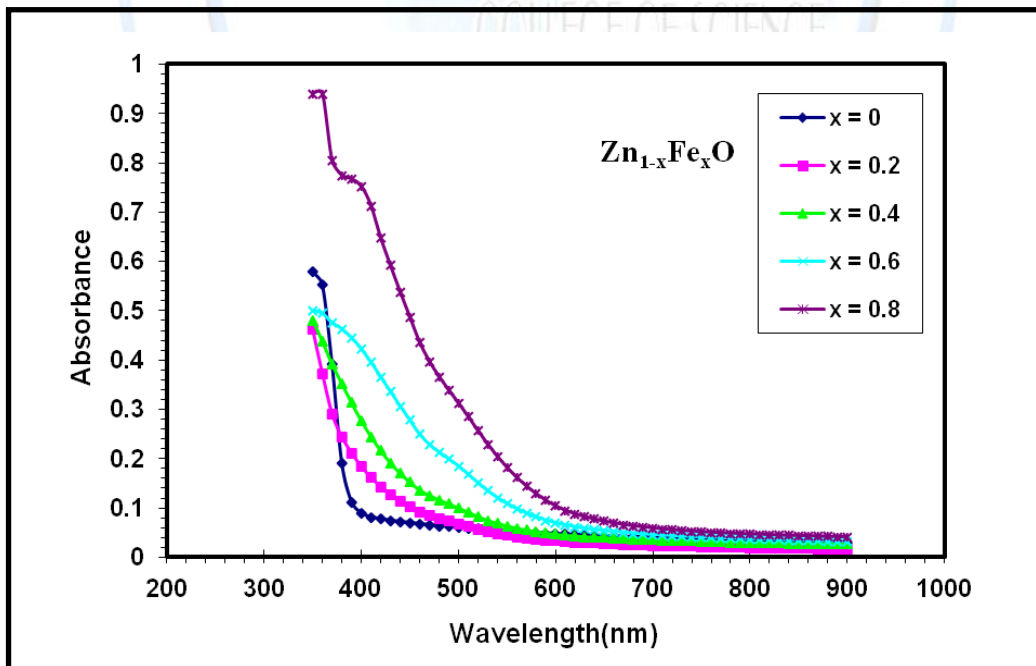
الشكل (2): يوضح تغير الامتصاصية لأغشية (Zn_{1-x}Fe_xO) بالنسب الحجمية (x = 0, 0.2, 0.4, 0.6, 0.8) .
